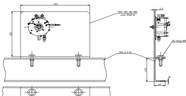
Hình 7. Thiết kế lắp đặt bộ hóa hơi, van điện từ, lọc LPG
