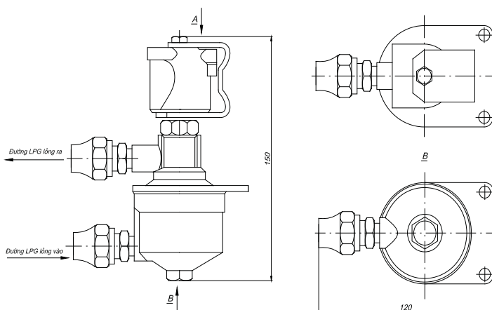
Hình 5. Kết cấu của van điện từ
