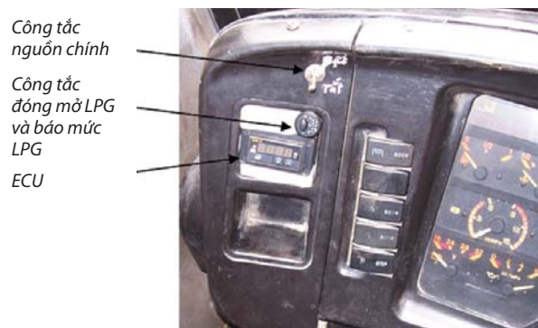
Hình 10. Ảnh chụp thực tế vị trí ECU và công tắc LPG khoang lái trên xe
