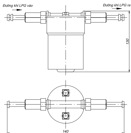
Hình 6. Kết cấu của bộ lọc LPG
