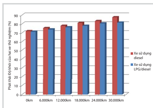
Hình 13. Phát thải độ khói của hai xe sau quãng đường thử nghiệm 30.000km
